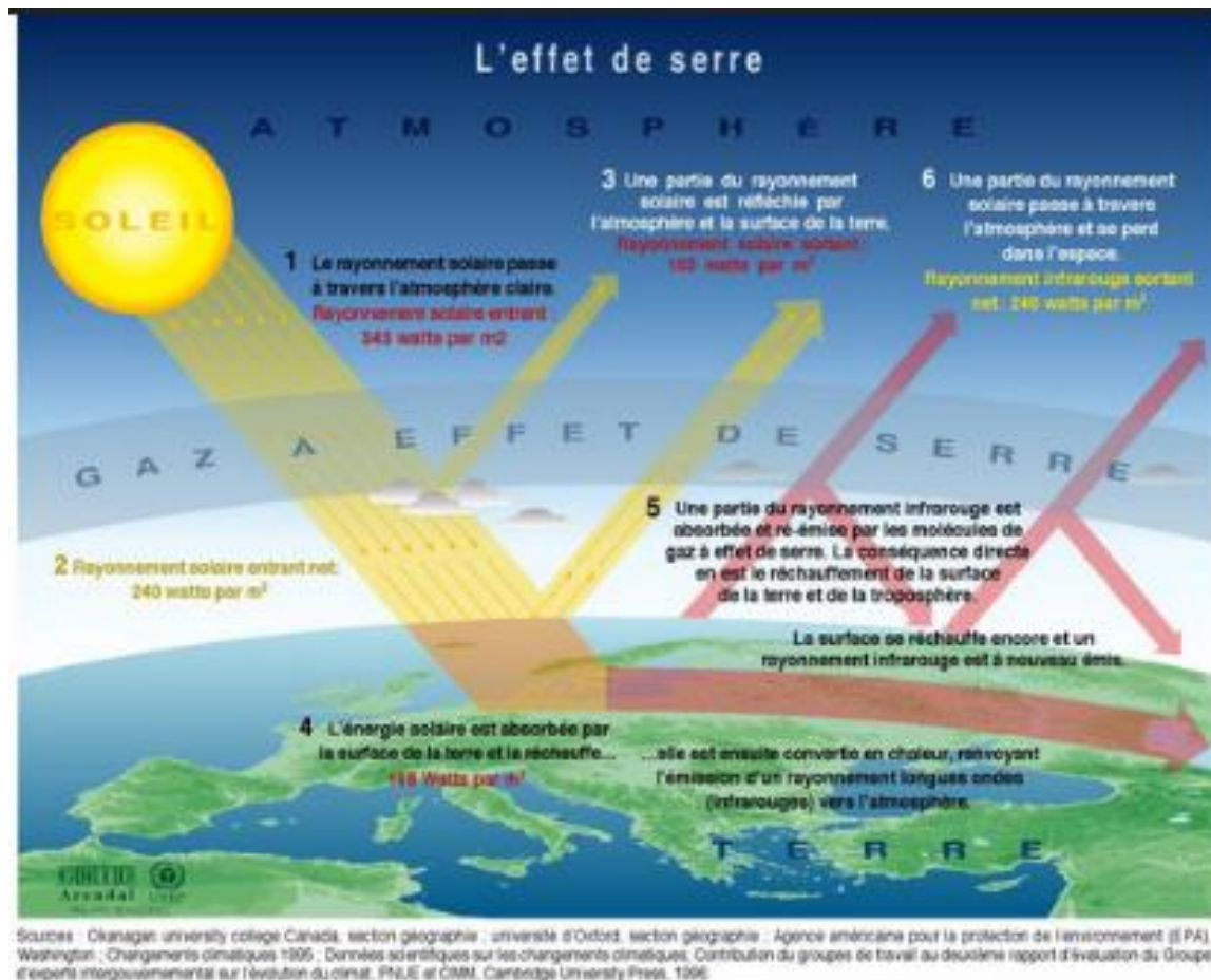
Figure 2 : Schéma de l'effet de serre
